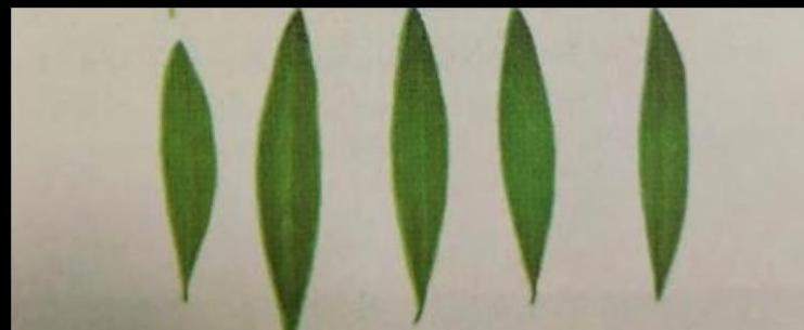
Figura 27.—Comparación de hojas de olivo, deficientes en potasio y boro, con hojas de olivos que han recibido aportes completos. Arriba: falta de potasio. Centro: falta de boro. Abajo: completo de nutrientes. (De H. T. Hartmann y J. G. Brown).
